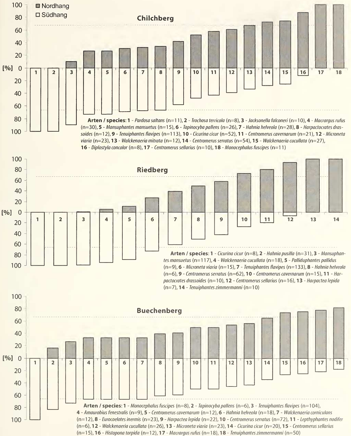
Abb. 11: Verteilung der Arten, mit mindestens 6 erfassten Individuen pro Untersuchungsgebiet, auf Süd- bzw. Nordhängen in Prozent; punktierte Linie = \frac{2}{3} der relativen Häufigkeit.
